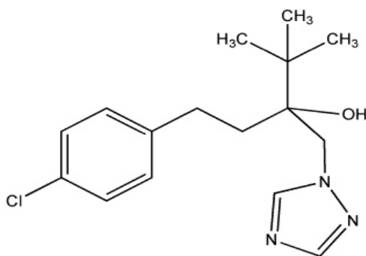
Rysunek 1. Nazwa chemiczna według IUPAC: ( RS )-1-(4-chlorofenilo)-4,4-dimetylo-3-(1 H , 1,2,4-triazol-1-ilometylo) pentan-3-ol
