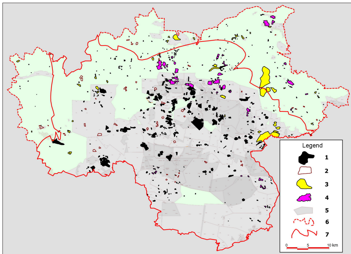
Ryc. 5. Rozmieszczenie wyrobisk surowców skalnych i zwałowisk w obszarze miejskim GZM na tle aktualnych obszarów górnictwa węglowego (perspektywa ważności koncesji 2020-2050). Objasnienia; 1 – wyrobiska powierzchniowe które obecnie są składowiskami dla KWK (zwałowiska), 2 – wyrobiska ilów i glin (glinianki), 3 – wyrobiska piasków i żwirów (piaskownie, żwirownie), 4 – wyrobiska skał zwięzłych (kamieniołomy), 5 – granica złóż na terenie GZM, 6 – granica GZM, 7 – granica GZW.
