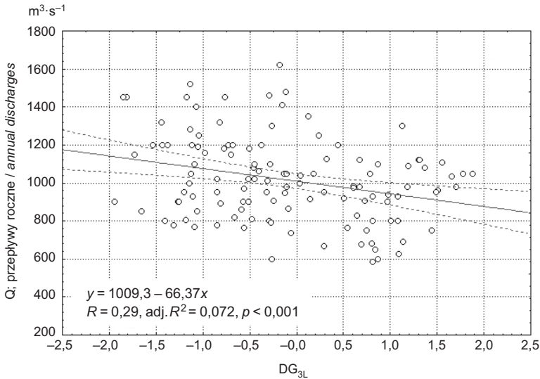
Ryc. 3. Przepływy roczne Wisły w Toruniu w funkcji wskaźnika \text{DG}_{3L} (1880-2000) Correlation between mean annual discharges of the Vistula at Toruń and the \text{DG}_{3L} index (1880-2000)
