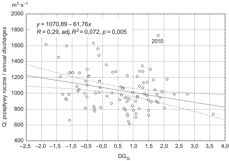
Ryc. 2. Przepływy roczne Wisły (profil Tczew) w funkcji wskaźnika \text{DG}_{3L} , charakteryzującego zmiany natężenia THC na Atlantyku Północnym (1921-2015). Oznaczono wartość odstającą (rok 2010)
