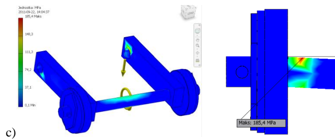
Rys. 13. Wyniki analizy MES otrzymanych naprężeń osi z kołami dla materiałów a) brzoza, b) brzoza, c) dąb
