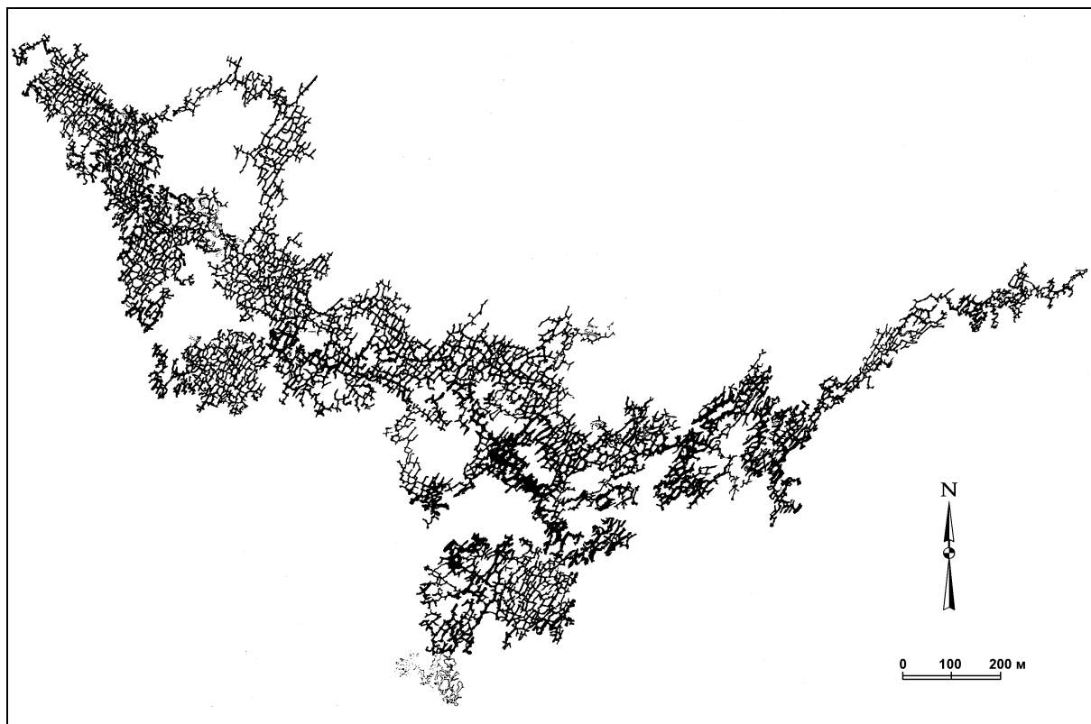
Ryc. 5. Plan odsłoniętej przez kamieniołom Kriwskij jaskini Popelushka (materiały Bukowińskiego Klubu Speleologicznego Troglodyta ).
