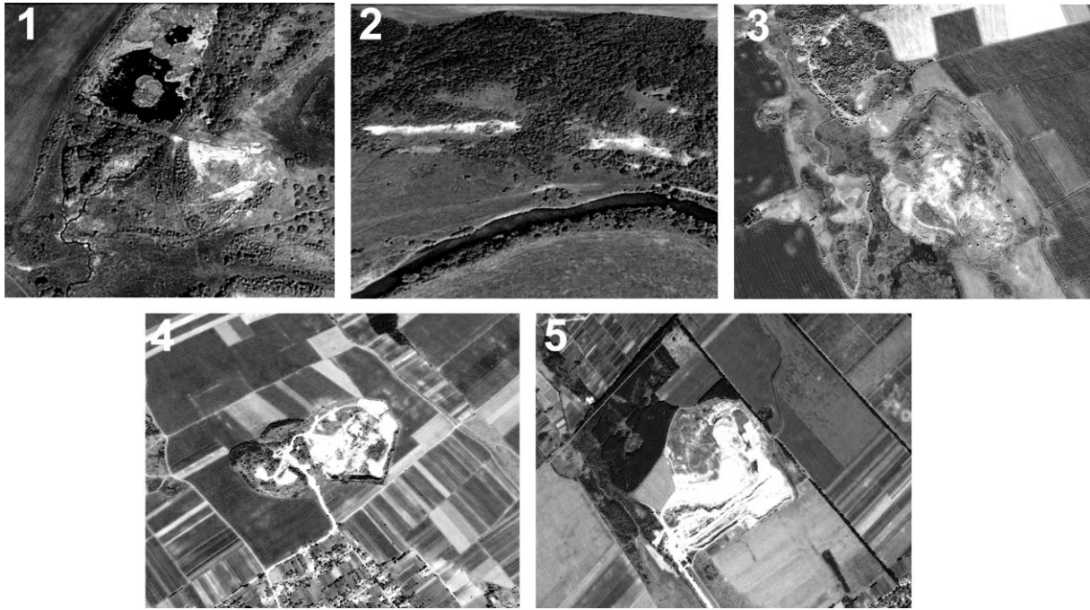
Ryc. 2. Widok z lotu ptaka opisywanych w artykule kamieniołomów gipsowych: 1 – kamieniołom Nagórzański, 2 – kamieniołom Zawaliwskij, 3 – kamieniołom Stalniweckij, 4 – kamieniołom Mamalyżskij, 5 – kamieniołom Kriwskij.
