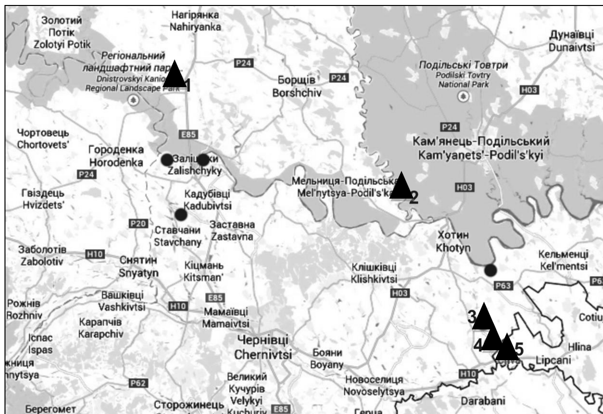
Рис. 1. Lokalizacja ważniejszych czynnych i nieczynnych kamieniołomów gipsowych w naddniestrzańskiej części Podola oraz na Bukowinie: czarne trójkąty – kamieniołomy opisane w artykule, czarne kropki – nie opisywane. 1 – kamieniołom Nagorzanskiy, 2 – kamieniołom Zawaliivskiy, 3 – kamieniołom Stalniwecki, 4 – kamieniołom Mamaizskiy, 5 – kamieniołom Krivskiy.
