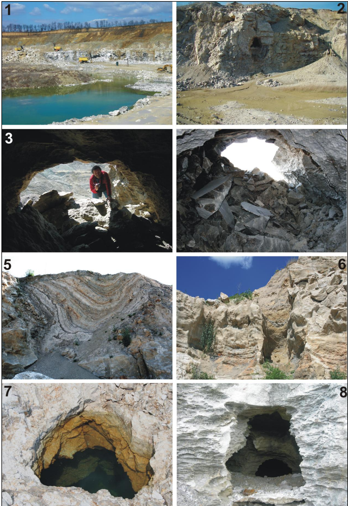
Ryc. 7. Formy krasowe odsłaniające się w ścianach i na dnie kamieniołomu Kriwskiego. Fig. 7. Karst forms exposing in the walls and on the bottom of the Krivskiy quarry.
