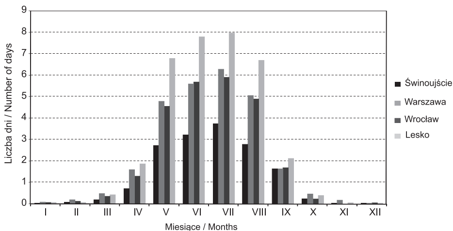
Ryc. 3. Roczny przebieg liczby dni z burzą na wybranych stacjach w latach 1949–2006 Fig. 3. The annual occurrence of days with a thunderstorm at selected stations during 1949–2006
