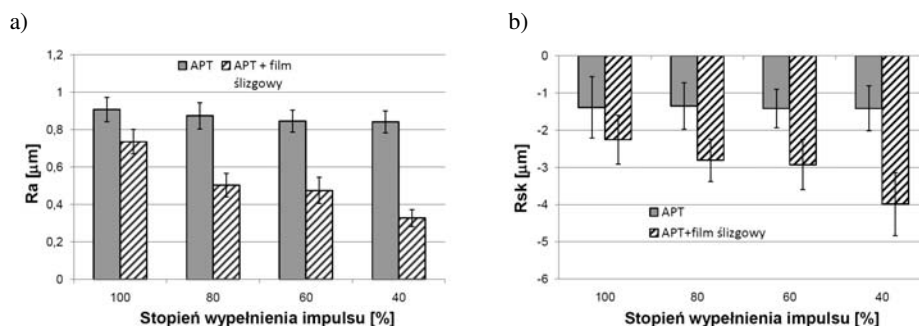
Rys. 3. Zmiana parametrów chropowatości powierzchni Ra (a) i Rsk (b) powłok tlenkowych wytworzonych metodą impulsową, stosując zmienne wypełnienie przebiegu prostokątnego prądu, przed i po współpracy tribologicznej z tworzywem PEEK/BG
